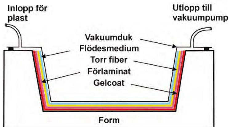
Schematisk beskrivning av vakuuminjicering.
