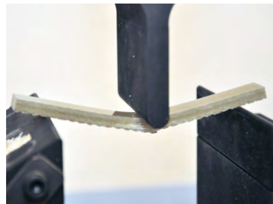
3-punkt böjprovning
