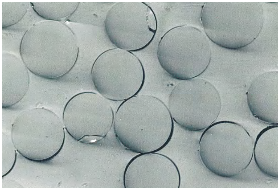
Släppning (debondning) mellan glasfiber och vinylester efter härdning. Släppningen beror på dålig vidhäftning mellan fibrerna och plasten vilket medför att plasten krymper ifrån fibern vid härdning.
