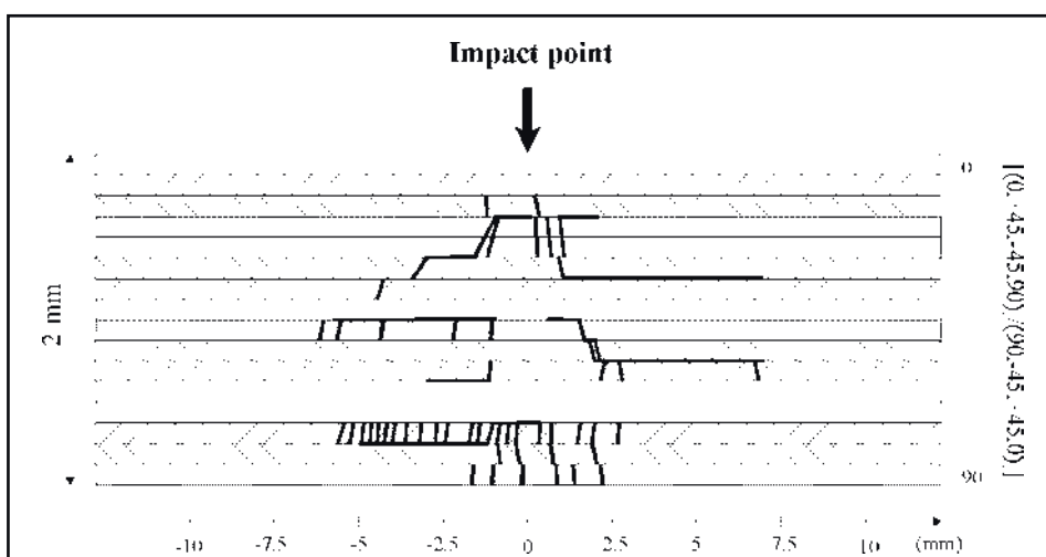
Schematisk beskrivning av slagskada i ett kvasi-isotrop laminat.
