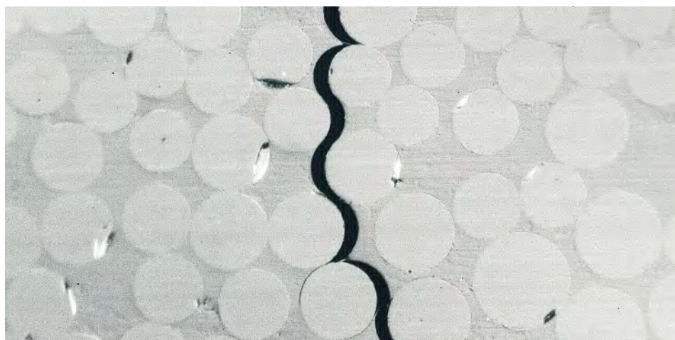
Transversell spricka i glasfiberarmerad vinylester. Sprickan uppstod vid låg töjning (< 0.2%) på grund av dålig vidhäftning mellan fibrerna och plasten.
