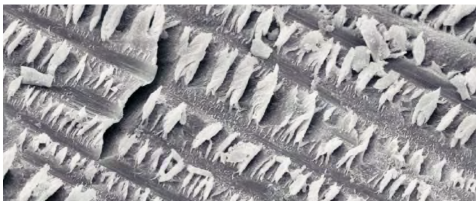
Brotttyta i kolfiberarmerad epoxi. Delamineringssprickan har tillväxt under skjuvbelastning.
