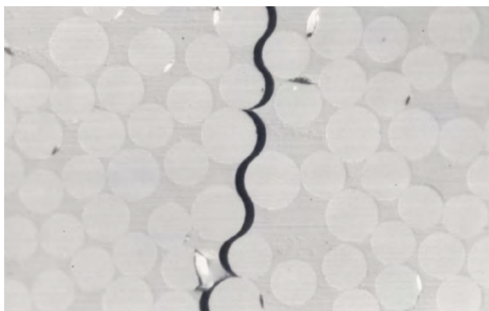
Transversell spricka i glasfiberarmerad vinylester. Sprickan uppstod vid låg töjning (< 0.2%) på grund av svagt fäste mellan fibrerna och plasten.
