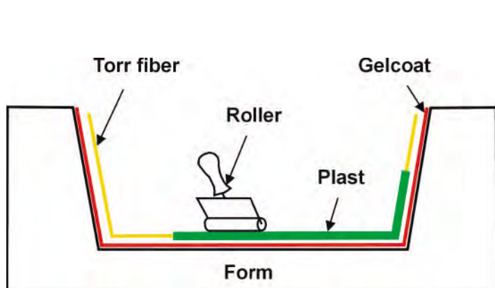
Schematisk beskrivning av handlaminering.
